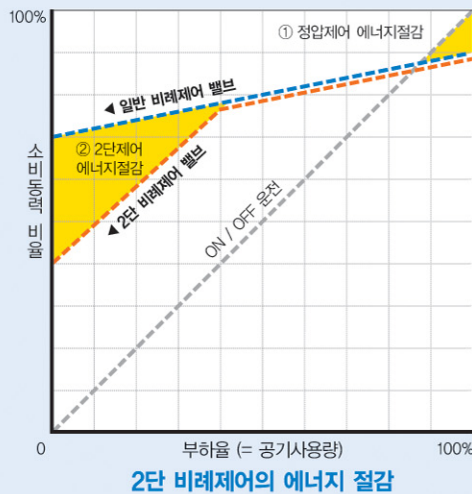
특허받은 2단계 에너지 절감형 석션밸브
