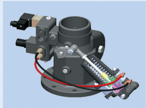
특허받은 2단계 에너지 절감형 석션밸브
