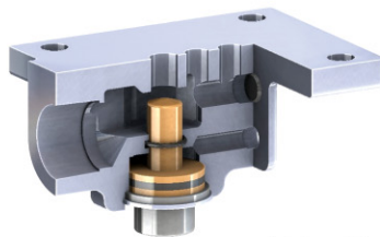
안정적 오일온도를 유지하는 오일 온도밸브
