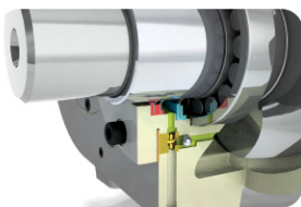
완벽한 누유방지를 위한 3단계 Shaft Sealing System
