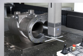
Screw Rotor 정밀측정
